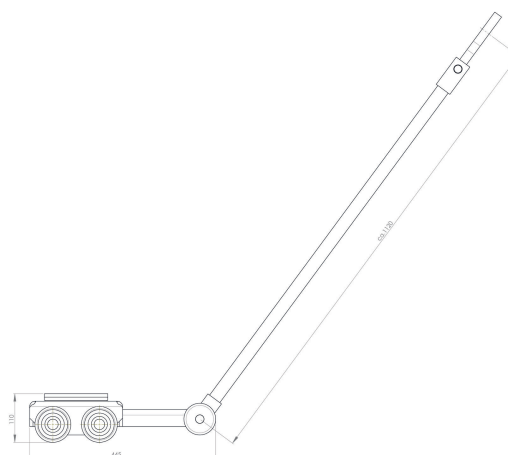
JLB 6 K | Art.No. 07 061 085-V | Seitenansicht | Side view
