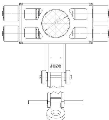
JLB 6 K | Art.No. 07 061 085-V | Draufsicht | Top view
